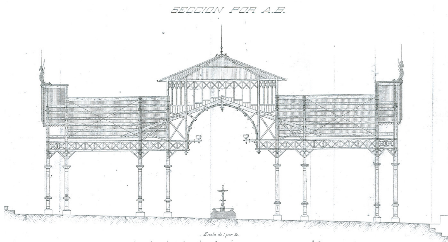
Alzado del proyecto de mercado público de Burjassot, proyectado en 1890.
