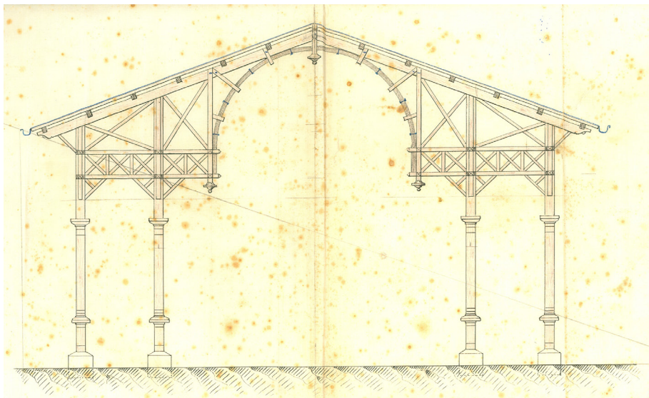
Sección de la peculiar estructura del Mercado Municipal, proyectado en 1890.
